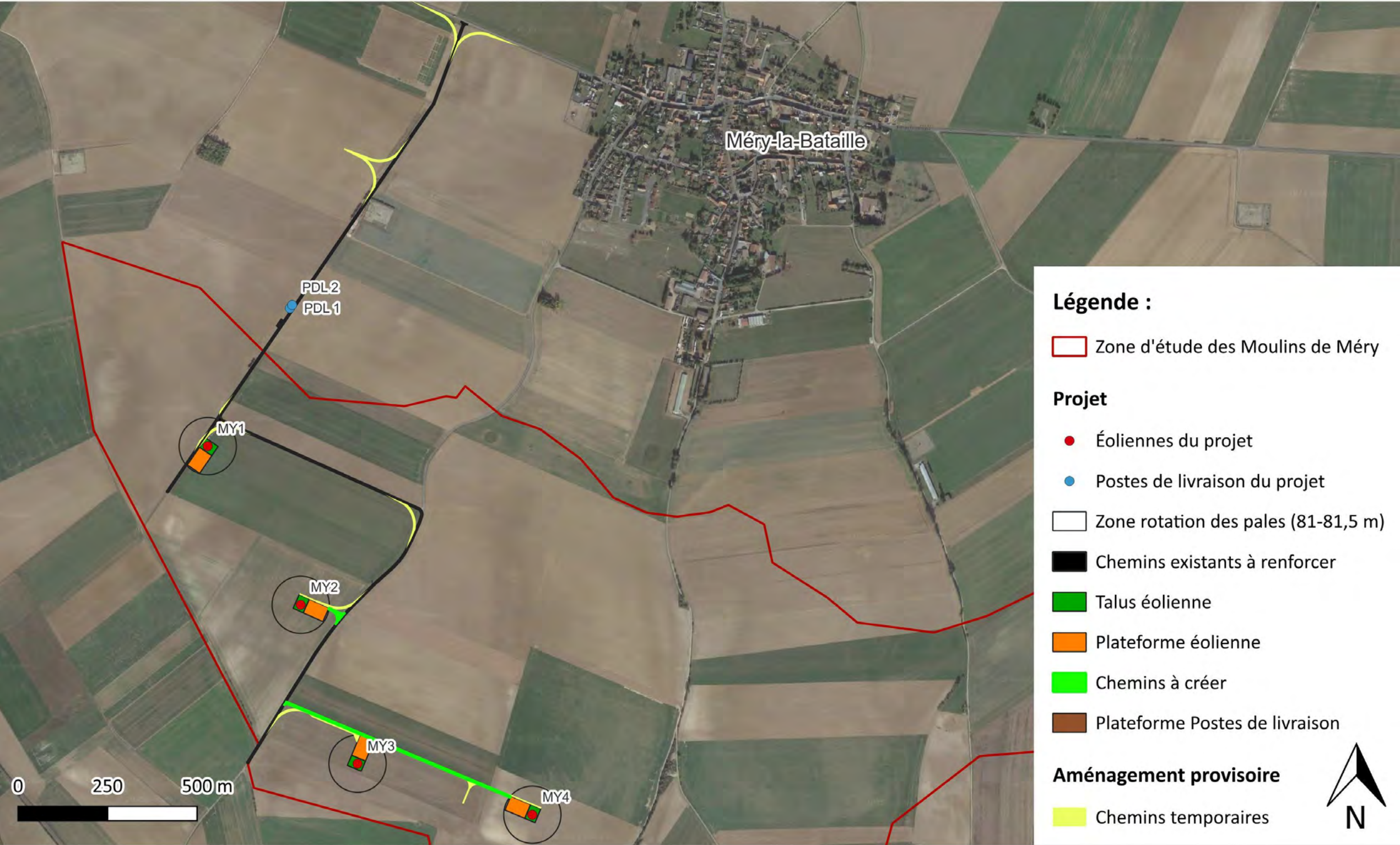
Carte 30 : Implantation prévisionnelle de la variante retenue pour le projet éolien des Moulins de Méry (60)
